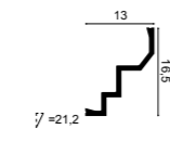
C300 200 x 16,5 x 13 cm Purotouch®
